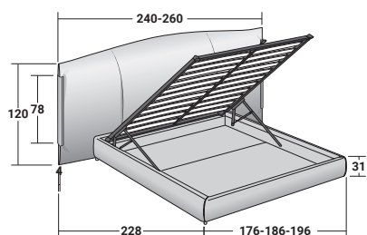
BASE CONTENITORE PIANO A DOGHE REGOLABILI
